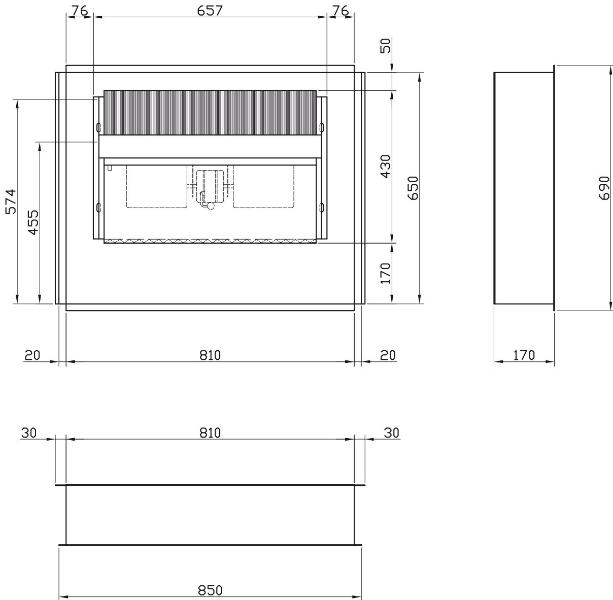
DIMA VENTILCONVETTORE Versione IN - Serie mini 2 FAN COIL UNITS Version IN - Series mini 2
